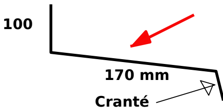
FAITIERE EN SOLIN ( ou Contre mur)
