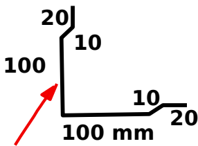
ANGLE BARDAGE EXTERIEUR
