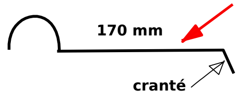
1/2 FAITIERE A BOUDN
