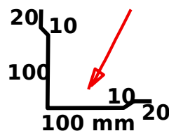
ANGLE BARDAGE INTERIEUR
